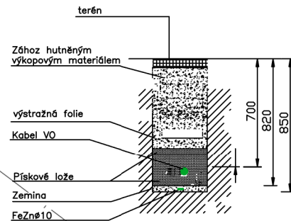
Typický řez trasou B - B
